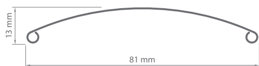
Secțiune transversală lamelă (C80)
